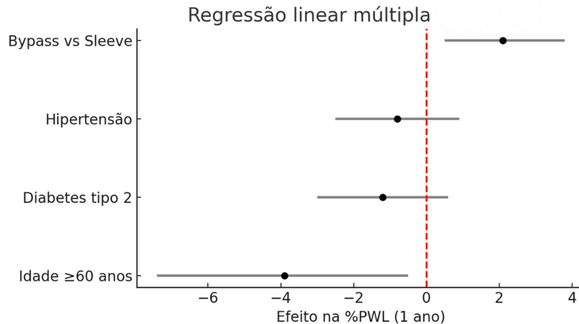
Regressão Linear Múltipla (Ajustada)
